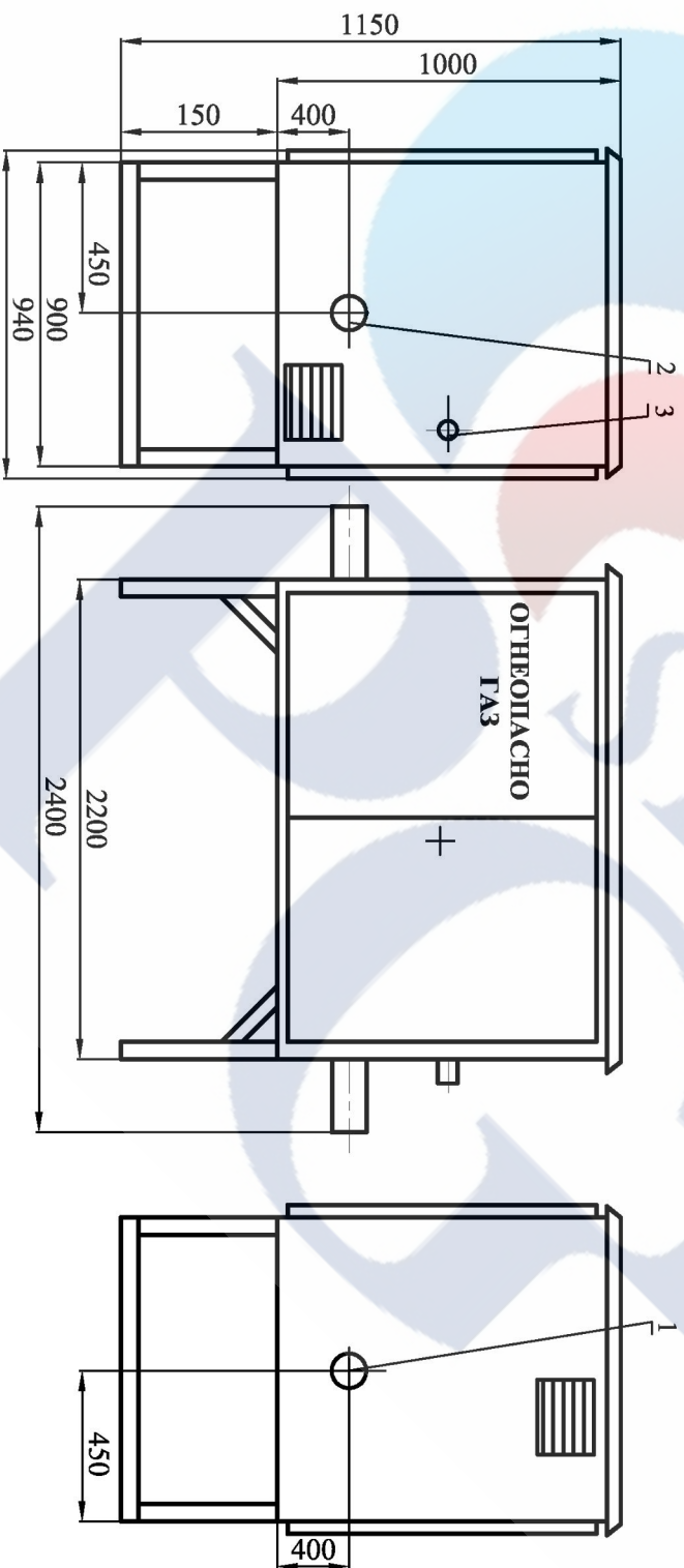
1 - Рвх. (Ду100); 2 - Рвых. (Ду100); 3 - продувочный патрубок (Ду20).
